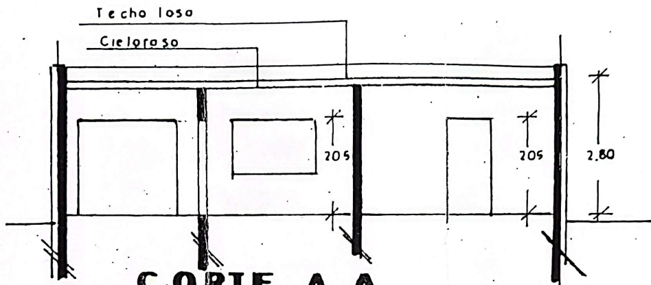
CORTE A-A
